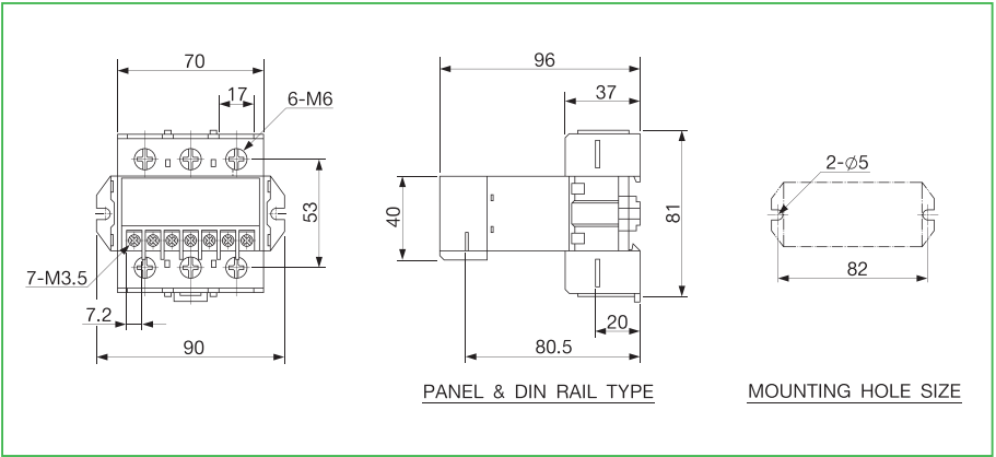
EOCR-DGT(接线端子型)
