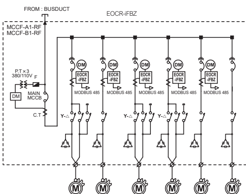
单线图
